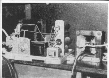
VOEDING VOOR: 450 V. ROOSTERSP. (regelb.) NEG.SP. -10 - -100 V. (regelb.) GLOEISP. 6V/3A
