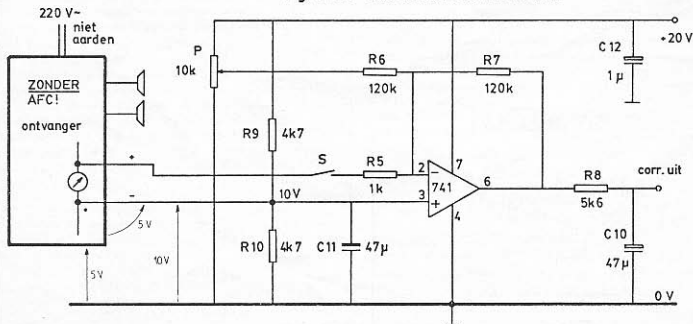
Fig. 4 DE STABILISATIESCHAKELING
