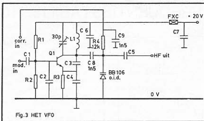
Fig. 3 HET VFO
