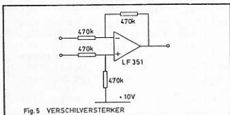
Fig. 5 VERSCHILVERSTERKER
