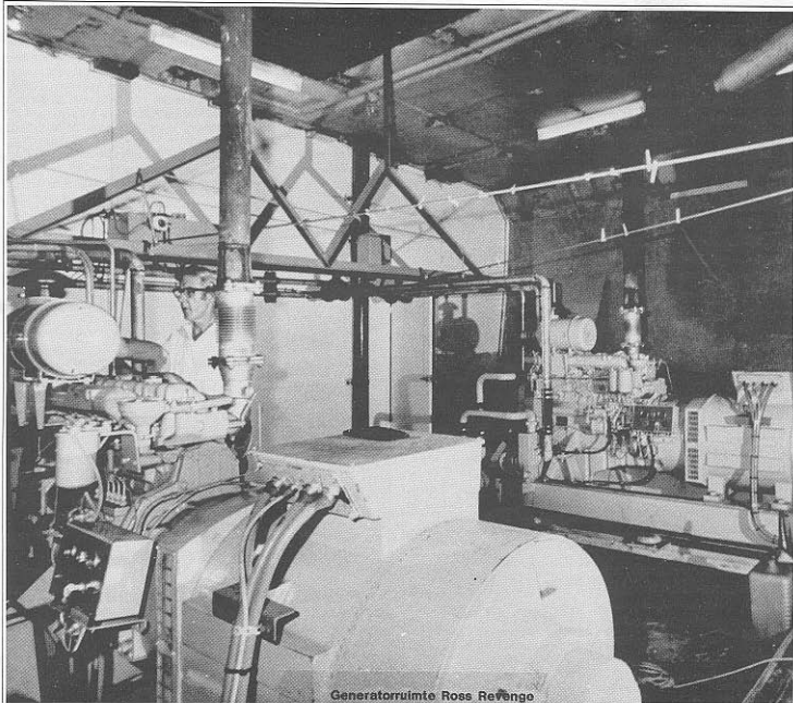
Generatruimte Ross Revenge
