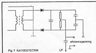
Fig. 7 RADIODETECTOR
